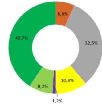
Gesamtdeutscher Energieträgermix 2022
